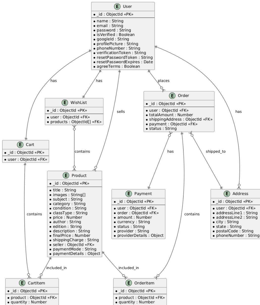
Figure: 1.7 – ER Diagram
